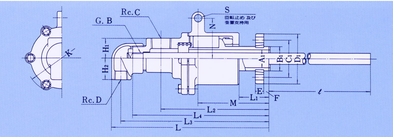
NCF Type 复式内管固定法兰安装式
