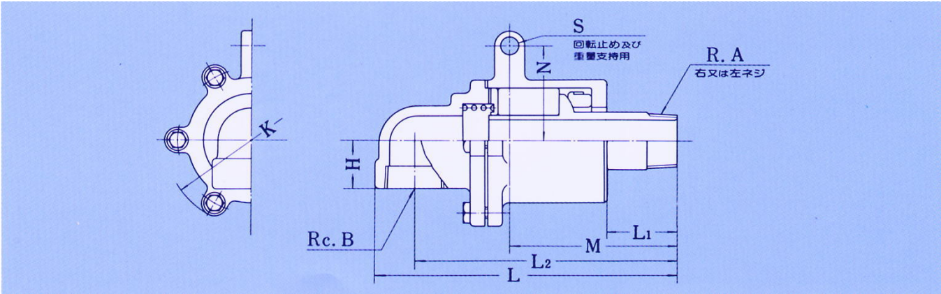
尺寸表 NCL Type 单式螺纹安装式
