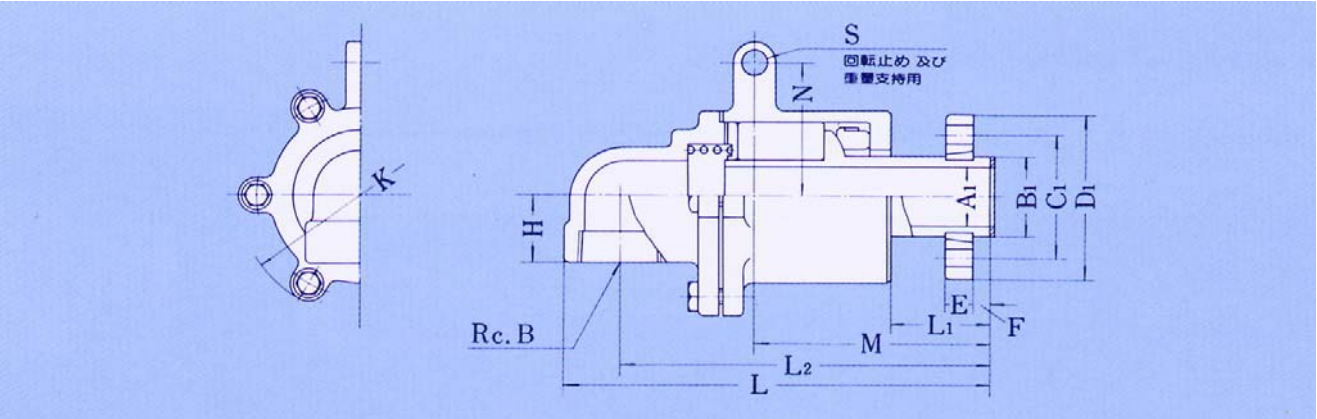
NCLF Type 单式法兰安装式
