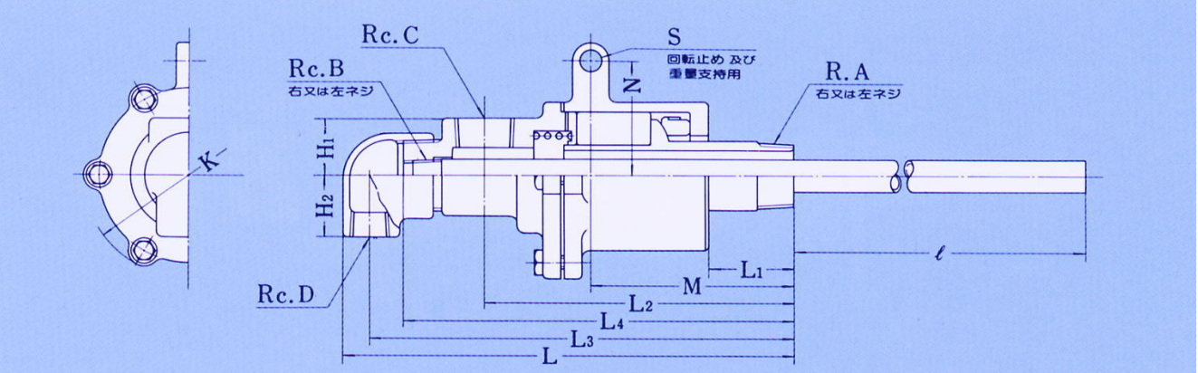
尺寸表 NC Type 复式内管固定螺纹安装式
