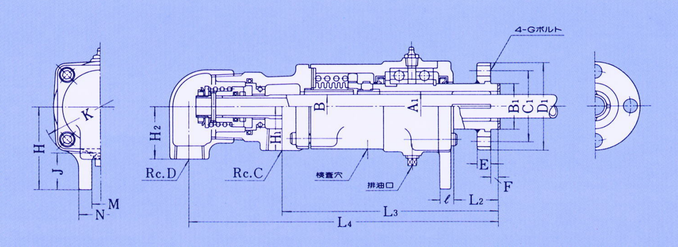
ACFW Type 复式内管旋转法兰安装式
