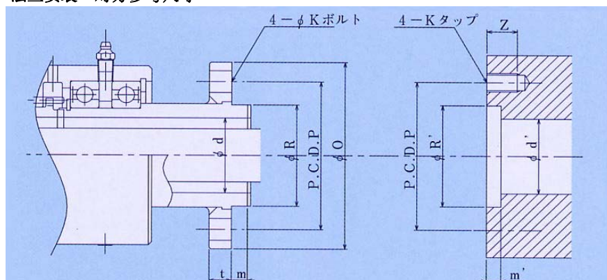
法兰安装 对方参考尺寸
