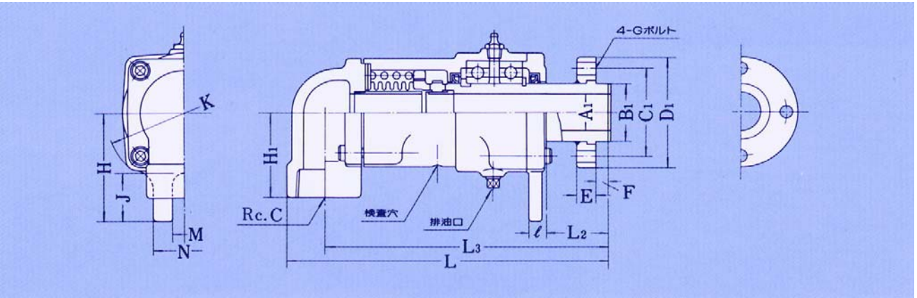
ACLF Type 单式法兰安装式
