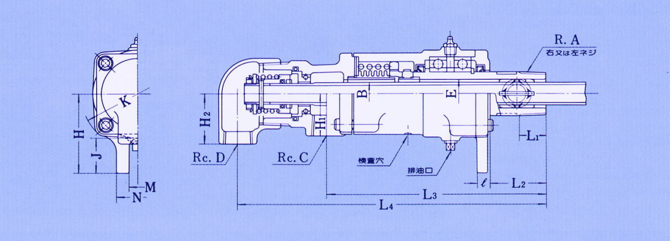
尺寸表 ACW Type 复式内管旋转螺纹安装式
