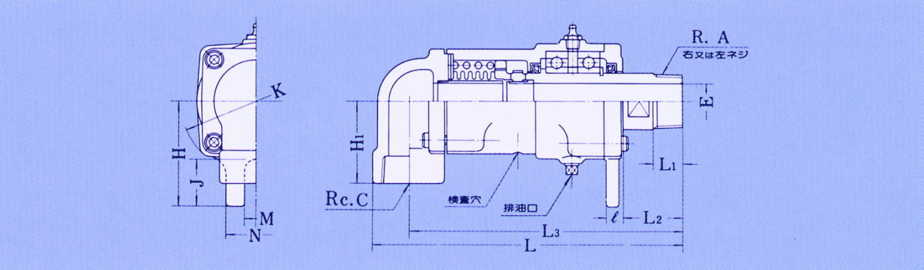
尺寸表 ACL Type 单式螺纹安装式
